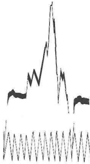
Spektrogram
