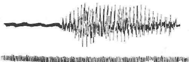
[şən] sözünün ossiloqramı 2
